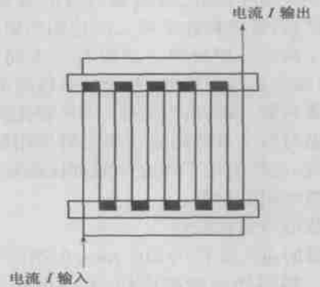
图6 加热电阻结构平面展开示意图
