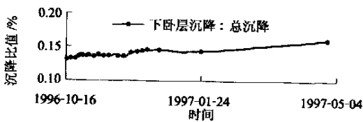
图3 下卧层沉降与总沉降比值变化曲线
