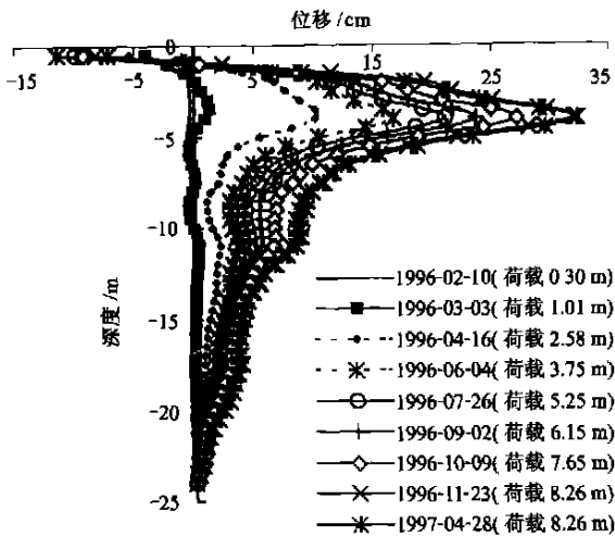
图7 路基水平位移变化过程线
