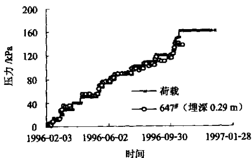
图 5 647# 土压力盒应力变化曲线
