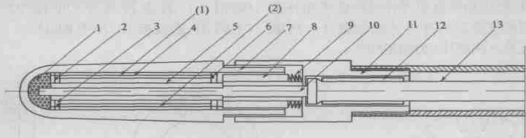
1—电极座;2—石墨板;3—绝缘板;4—石墨棒;5—绝缘套;6—联结板;7—外壳; 8—压环;9—压簧;10—电极杆;11—接头;12—绝缘套;13—压杆;(1)、(2)—石墨棒 图7 热熔器新式结构示意图
