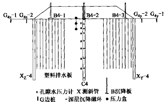
图 1 4 # 断面的观测元件布置示意图
