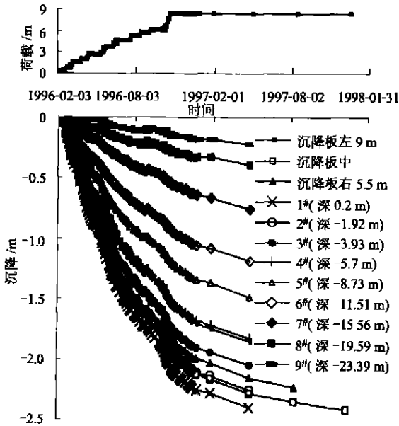
图2 4#断面 P-t-s 曲线
